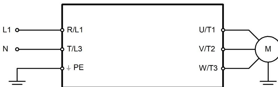
Подключение силовых клемм для моделей LCI-GY/PY-3
