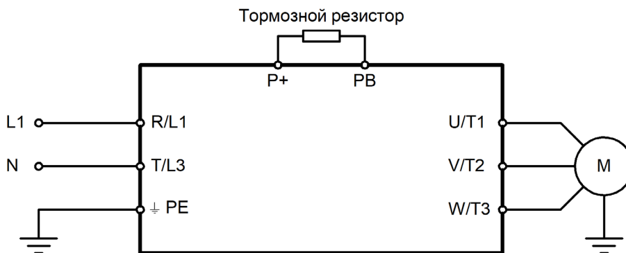
Подключение силовых клемм для моделей LCI-GY/PY-2(B)
