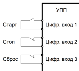
Четырехпроводное подключение
