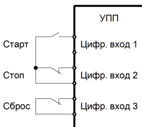
Трехпроводное подключение
